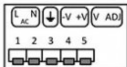
Схема подключения к электросети
